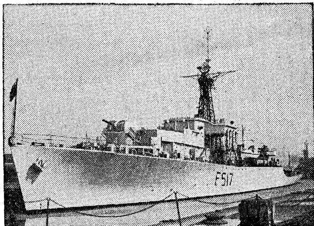
La fragata "Loch Morlich", recientemente cedida a la Marina neozelandesa, con el nuevo nombre de "Tutira". Desplaza 1.435 toneladas y desarrolla una velocidad de 19'5 nudos.—(Calpe)
