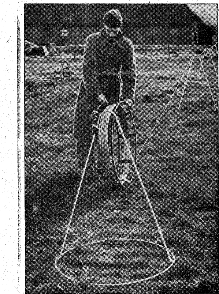
Para evitar que el ganado consuma los pastos en cantidad superior a la que necesita, se acotan los prados con cables conductores de electricidad, que limitan las superficies. La colocación es sencilla y rápida y los resultados, infalibles.—(Calpe)
