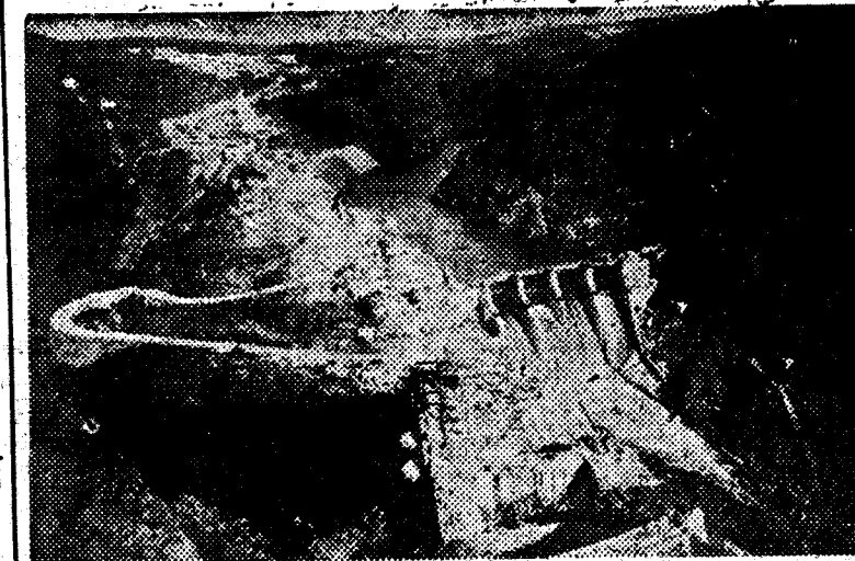
Una visita general del Salto del Castro, que ha sido inaugurado por Su Excelencia el Jefe del Estado. El embalse alcanza dieciocho kilómetros de longitud, con una capacidad total de treinta y ocho millones de metros cúbicos. La potencia es de 79,800 Kw., y su producción anual de 320 millones de kwh.
