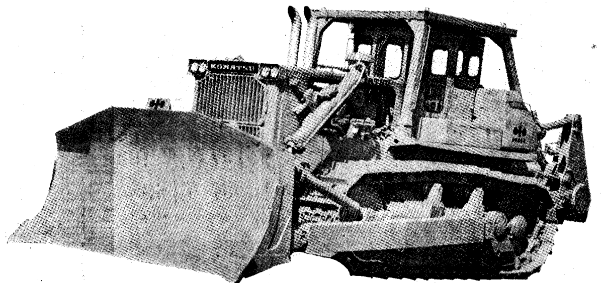
D455 A Bulldozer, Potencia neta al volante: 620 HP. (Dn) a 2.000 R.p.m. Peso en orden de trabajo: 78.410 Kgs.
