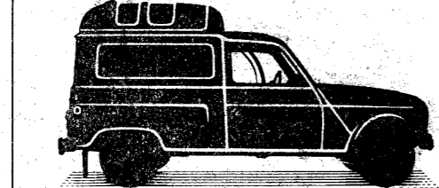
Sobreelevada Carga 425 kg. Altura útil 1,307 m. Volumen útil de carga 2,08 m 3
