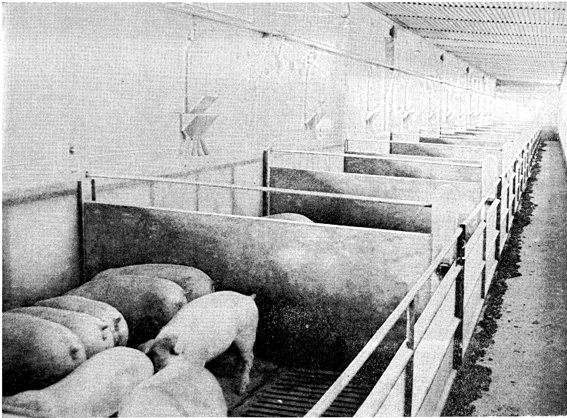
Una de las más recientes instalaciones gerundenses con equipos IBO, en una moderna granja de Crespiá, una nueva experiencia de las muchas adquiridas por IBO en nuestros comarcas.
