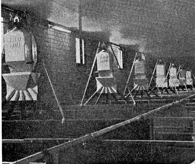
Modelo IBO-Split para comedero largo o atravesado, sistema dosificado por peso húmedo. Obsérvese cómo las placas de protección de los tubos de bajada tienen también la utilidad de servir de pared entre corrales.
