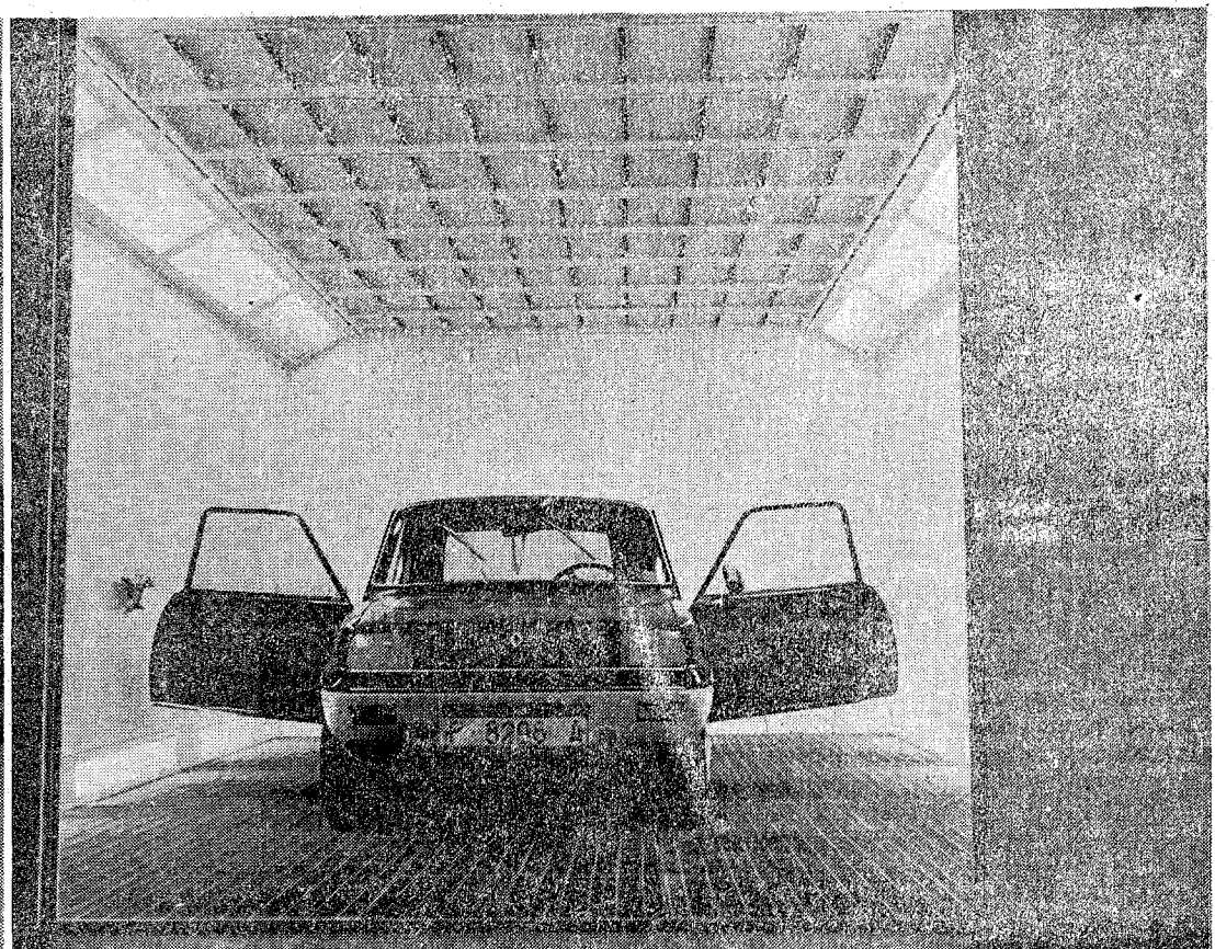
CABINA - HORNO BLACKHAWK, INSTALADA EN TALLERES ROME, S. L., C/. EMILIO GRAHIT, 73, DE GIRONA.
