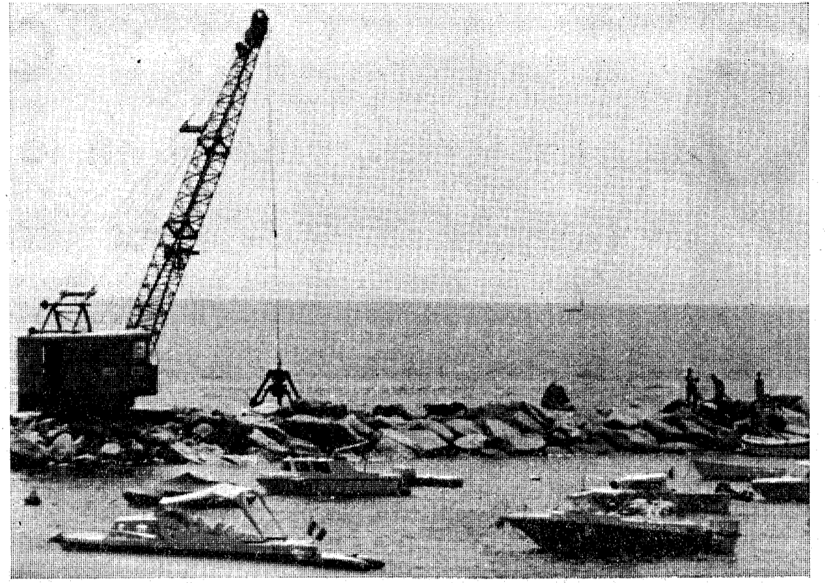
Las obras de defensa de la playa de Sant Antoni siguen a buen ritmo. (Foto Pablito)
