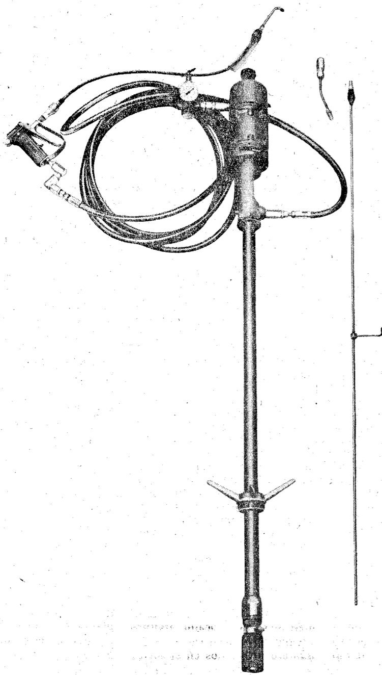
Equipo de pulverización para el tratamiento anticorrosivo Dinitrol, compuesto por bomba de alta presión Cairlese, pistola, boquillas de pulverización y varilla larga.
