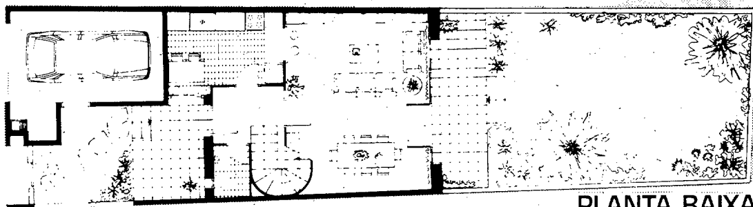
PLANTA BAIXA
