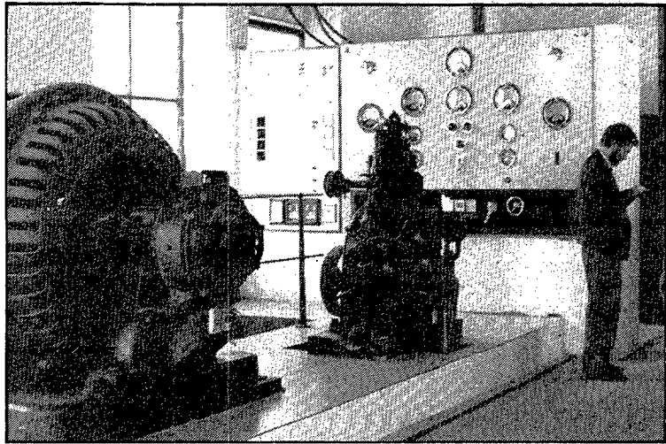
A l'esquerra, una de les turbines instal·lades el 1921 i, a la dreta, la nova abans de ser col·locada. La necessitat d'obra d'infraestructura per a la nova és molt inferior com es comprova pel seu tamany.
