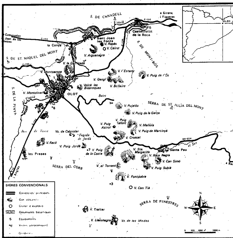
La zona volcànica de la Garrotxa, amb una trentena de cons volcànics.
