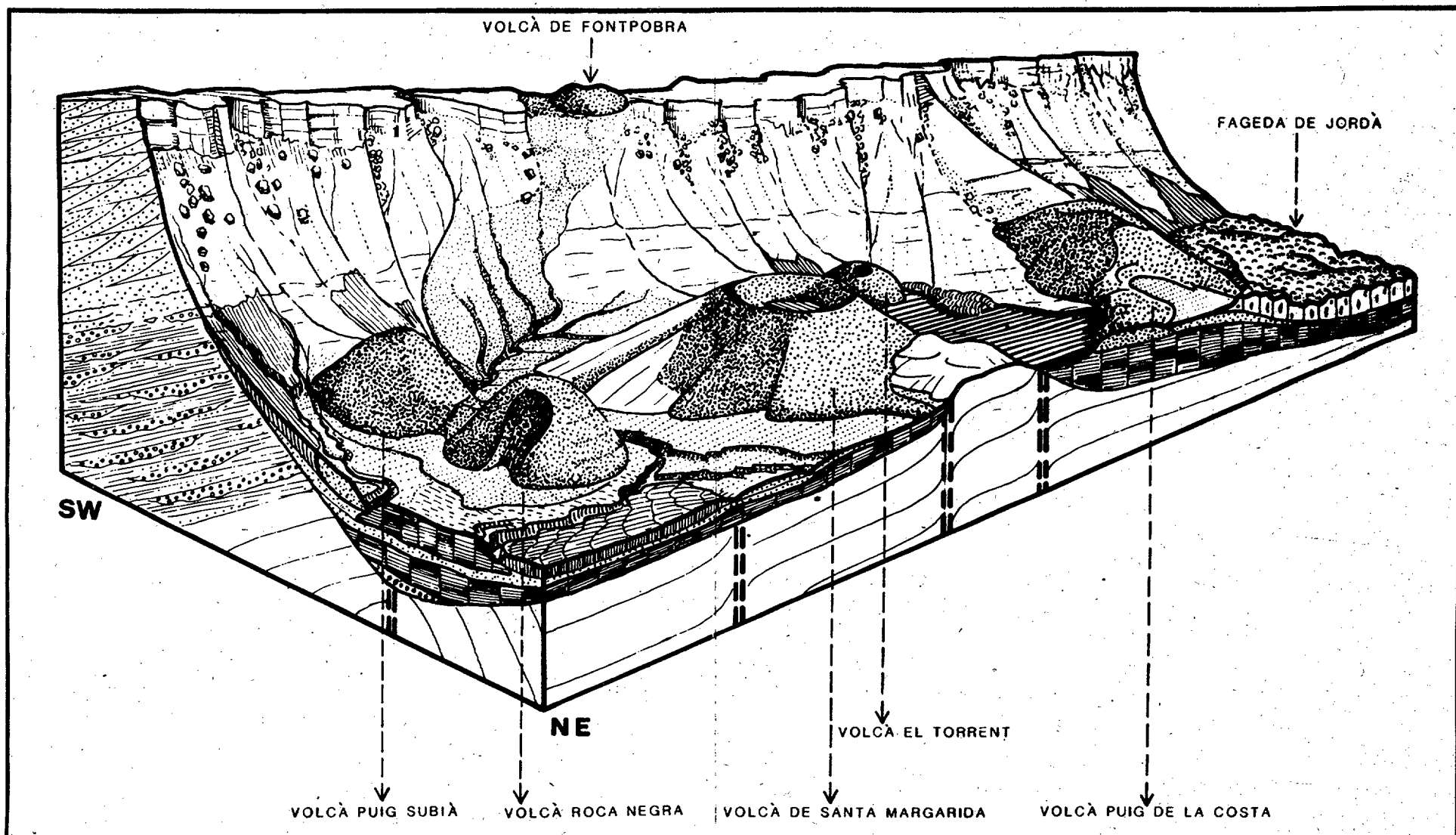
Tall transversal d'una de les parts de la zona volcànica de la Garrotxa.
