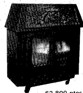
62.800 ptes. Estufa de llenya SALGUEDA-ISSA mod. Kaminet 12500 Kcal/h., sortida fums superio- rior + posterior 120, 890x700x450, 35 kg.
