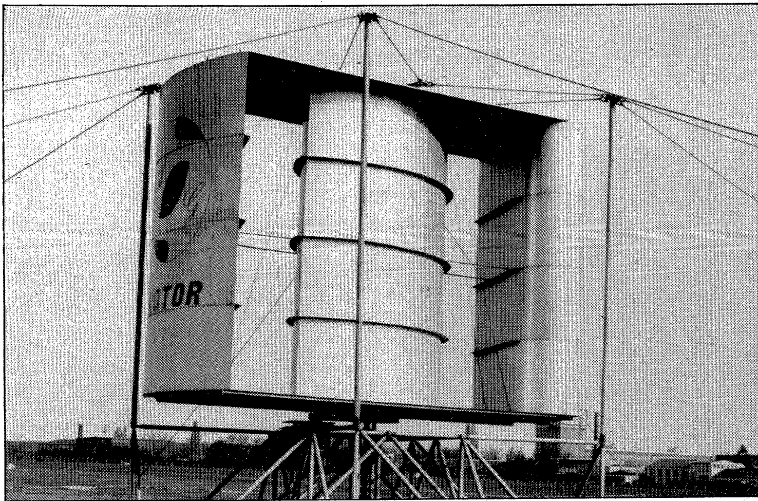
El vent és aprofitat per a la producció d'electricitat.
