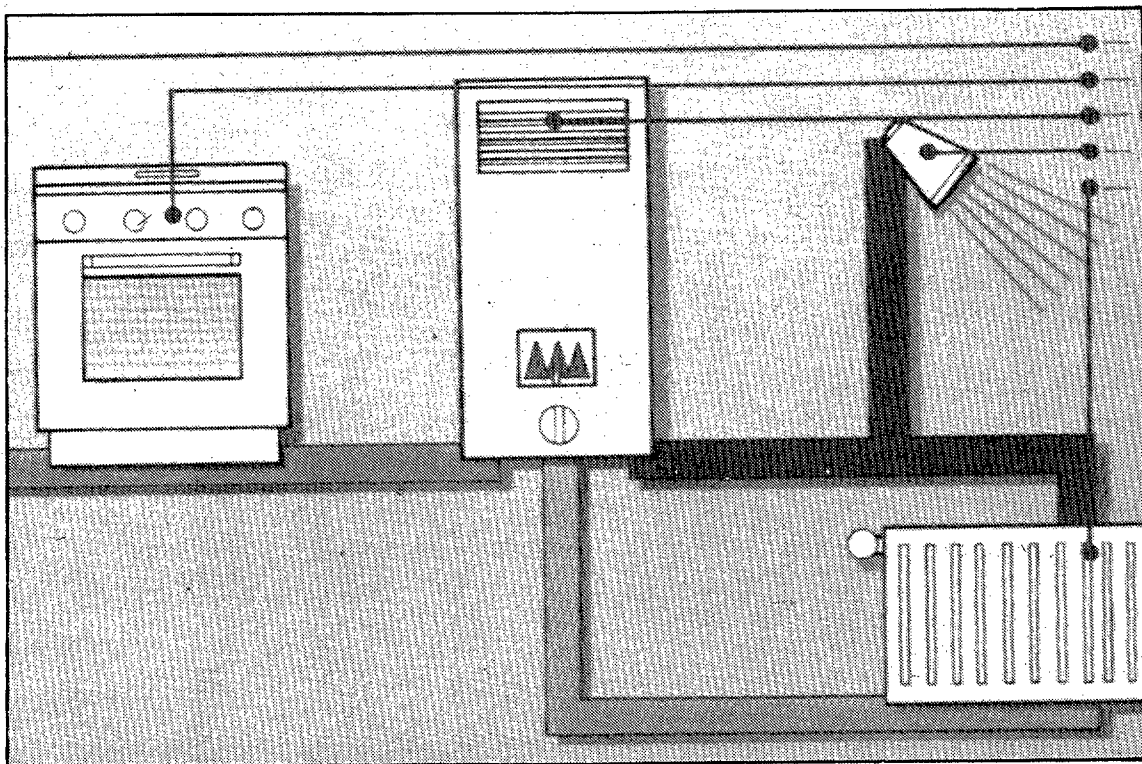
Una instal·lació de gas propà permet l'aprofitament per a tres usos, cuina, aigua calenta i calefacció.
