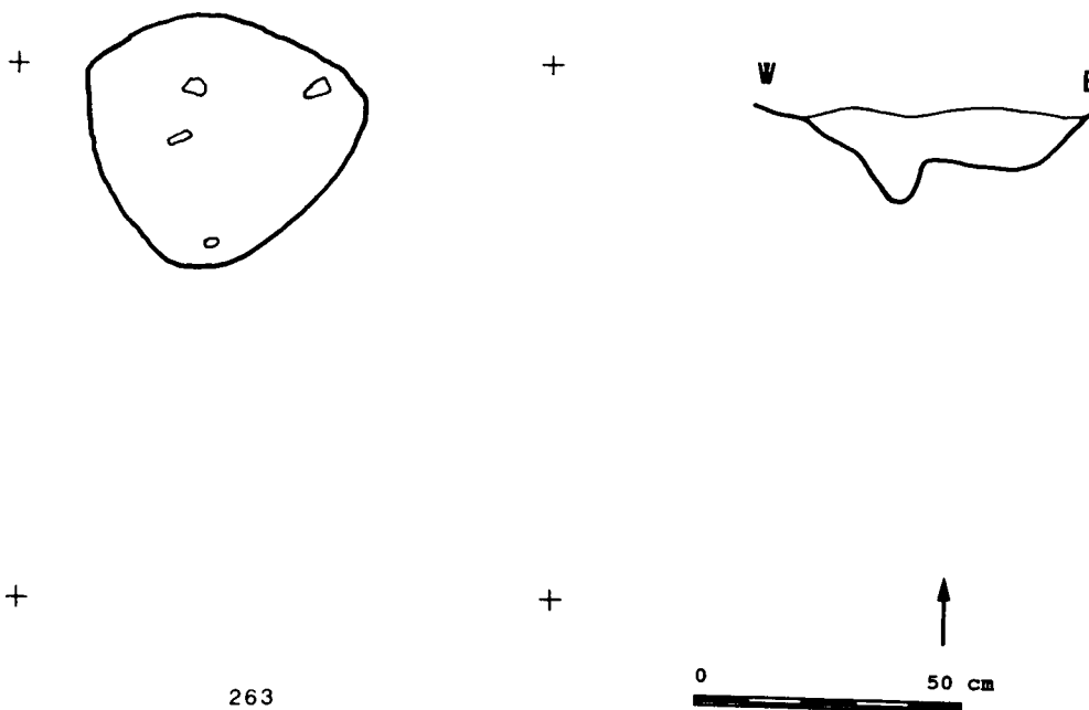
Fig. 12.- Planta i secció de la fossa del Nivell Arqueològic H-2. Quadre 263,555.
