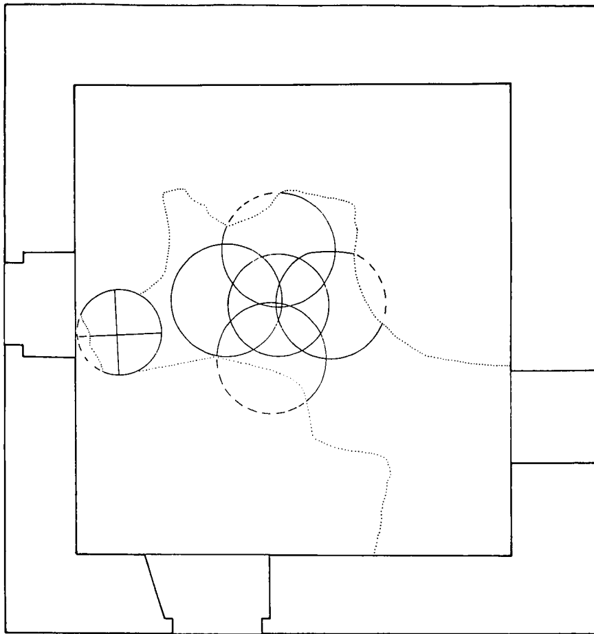
PLANTA DE LA TORRE Paviment de palets de riu formant cercles secants E. 1:50
