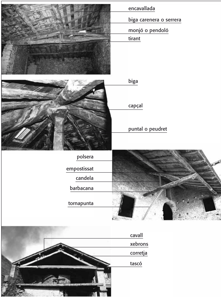
Figura 6.8. Elements constructius dels sostres
