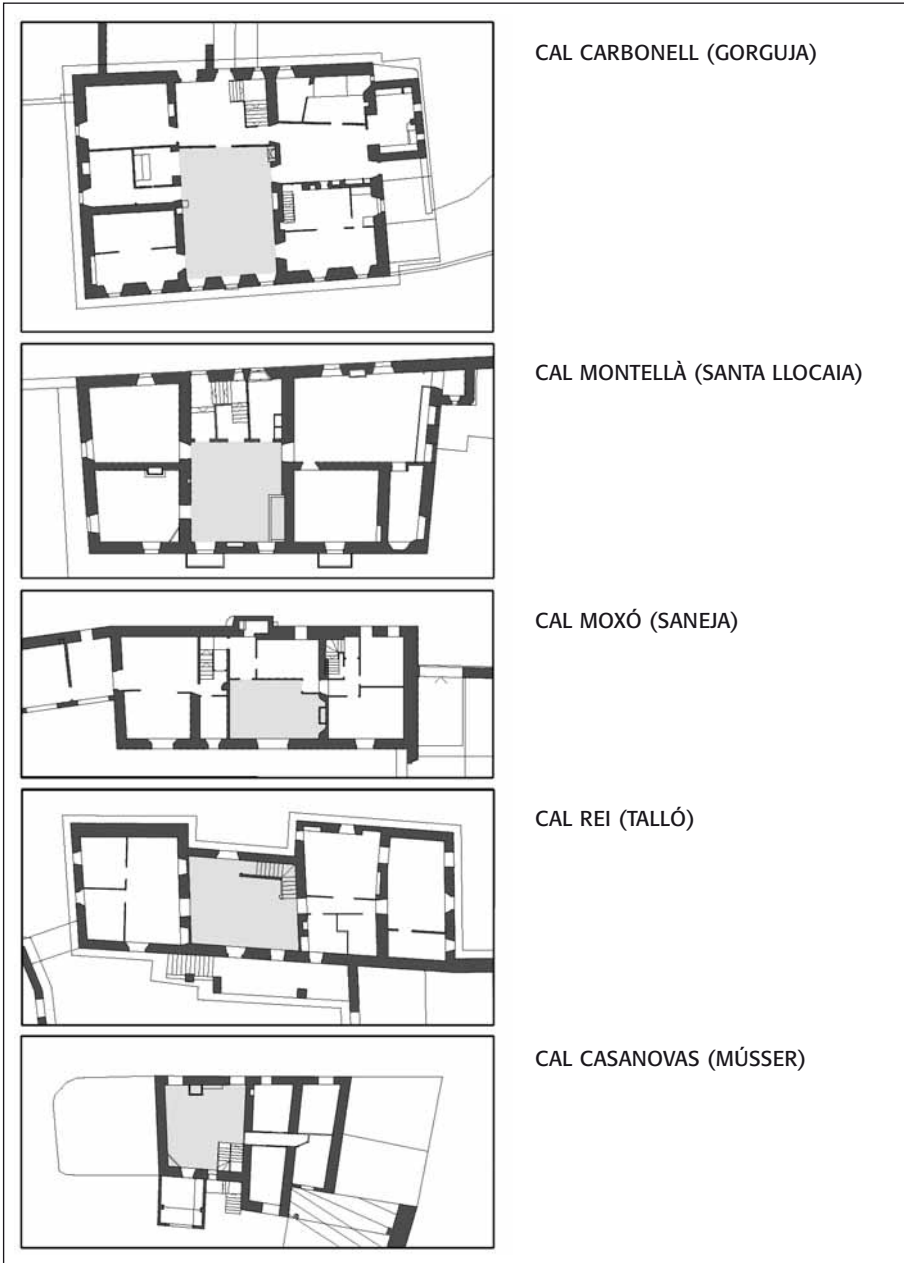
Figura 6.6. La distribució de la casa
