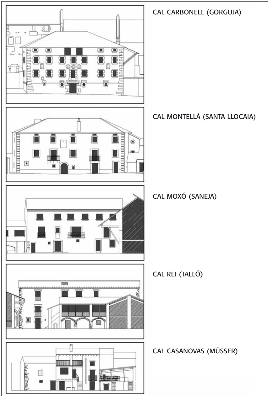
Figura 6.7. Alçats principals dels habitatges
