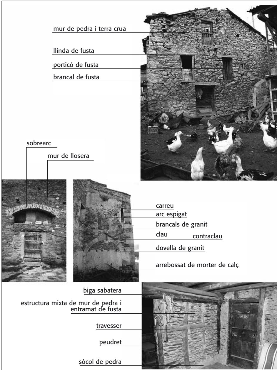
Figura 6.9. Elements constructius dels tancaments verticals
