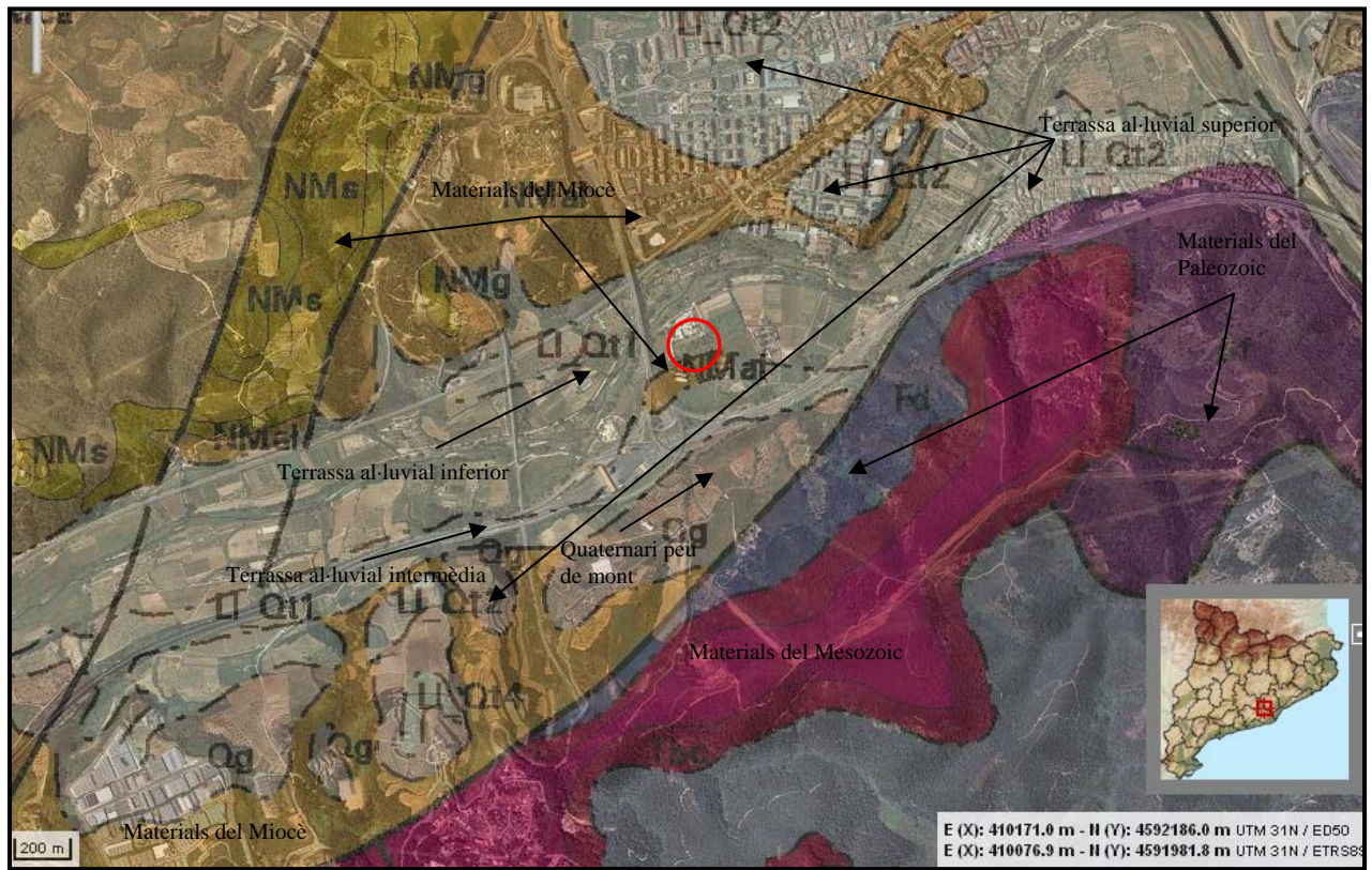
Fig. 2: Mapa geològic
