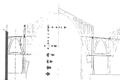
Arcs equilibrats
