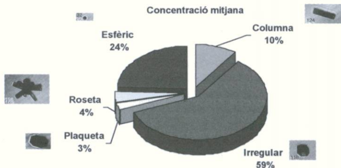
Diagrama 5. Proporcions dels cristalls de gel utilitzades pel tercer cas. Dades de la campanya EMERALD.
