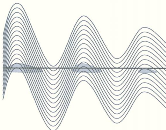
Diagrama 6. Representació dels nivells, les trajectòries de l'avió i de les simulacions. Línia gruixuda trajectòria de l'avió, línies fines trajectòries del model, zones grises nivells.
