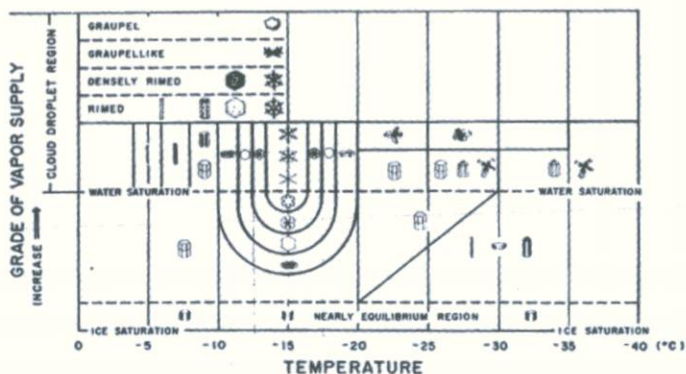
Diagrama 3. de Magono i Lee (1966) per la forma dels cristalls de gel en un gràfic de Humitat versus Temperatura
