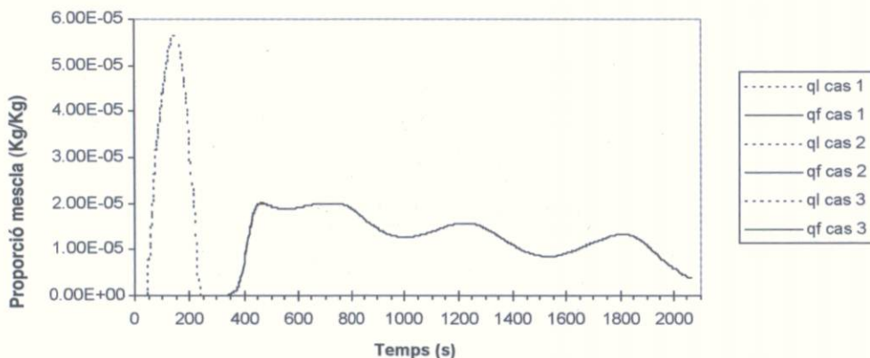
Diagrama 8. Gràfic de la quantitat d'aigua líquida i gelada segons les simulacions. Representa l'aigua líquida i amb l'aigua gelada. Els casos es refereixen als casos de diferents formes pels cristalls de gel.
