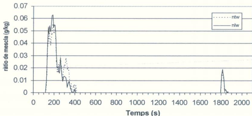
Diagrama 7. Gràfic de la quantitat total d'aigua (línia discontinua) i de l'aigua líquida (línia contínua) versus el temps de simulació.
