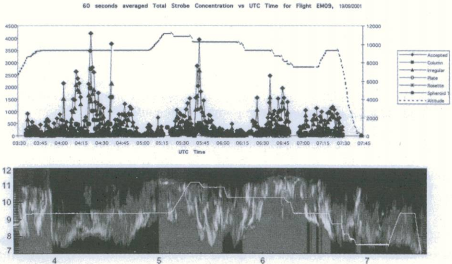
Diagrama10, Gràfic de la concentració de partícules i imatge Lidar en blanc i negre pel vol EM09. En la imatge a), la línia discontinua representa l'altitud de l'Egrett, les altres línies són diferents concentracions. En la imatge b) del Lidar tenim indicat amb la línia blanca l'altitud de l'Egrett les zones més clares són on tenim la més alta reflectivitat. (Imatges Lidar per Witheway i Cook)
