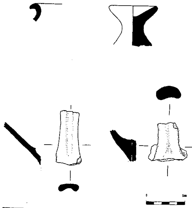
Fig.7 Ceràmica ibèrica. Formes
