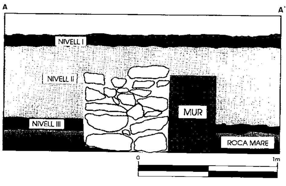
Fig. 5. Secció sector Est, àrea excavada poblada ibèrica
