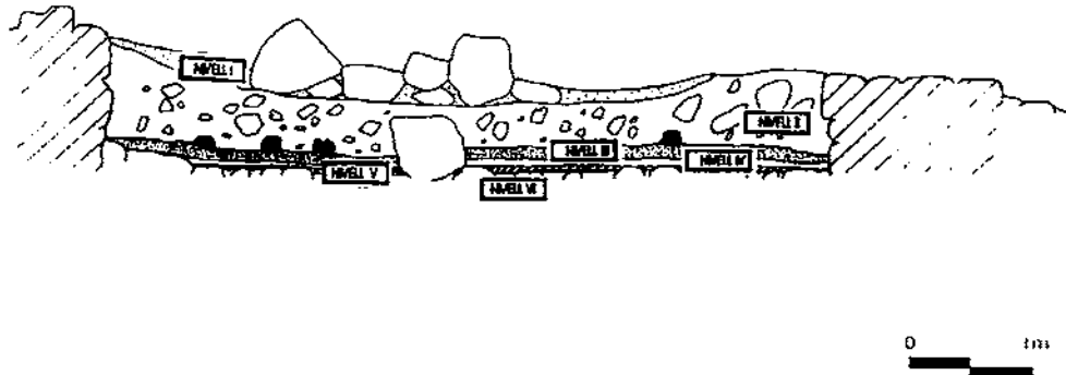
Fig. 6 Secció àrea excavada de la torre
