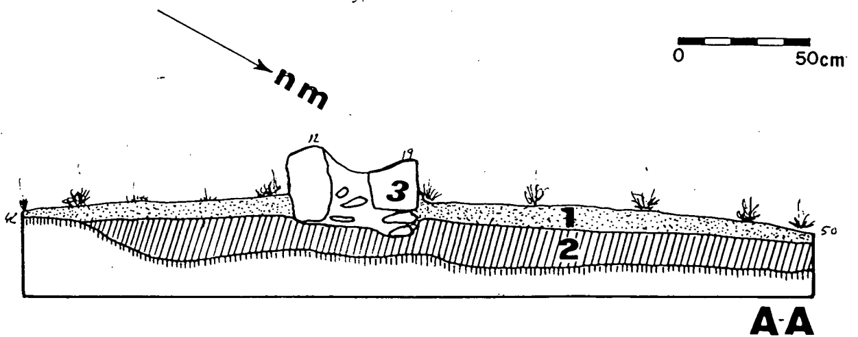
Planta i secció del sondeig B de Can Comelles. 1. Terra vegetal. 2. Terra estèril 3. restes d'un mur.
