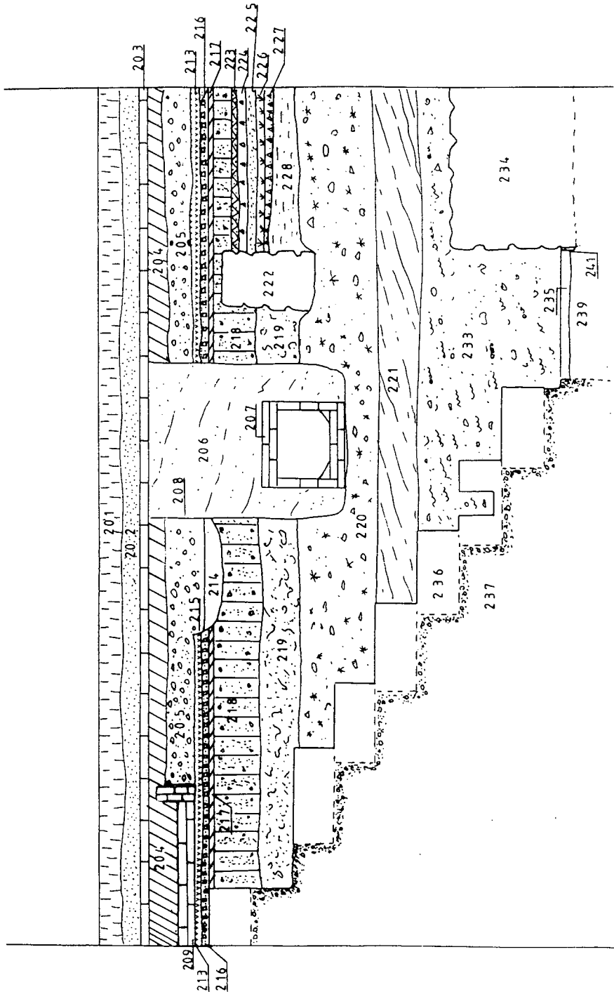
SECCIO F-F
