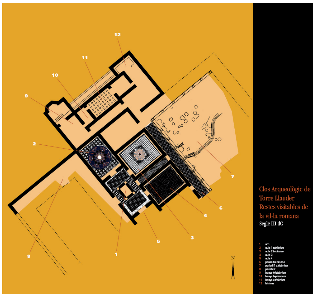
Figura 1. Planta general de la pars urbana de la vil·la
