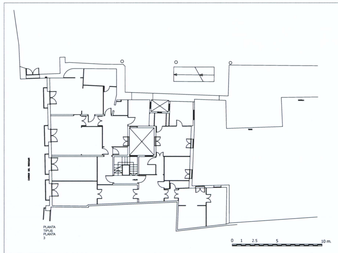
Planta del tercer pis de l'edifici
