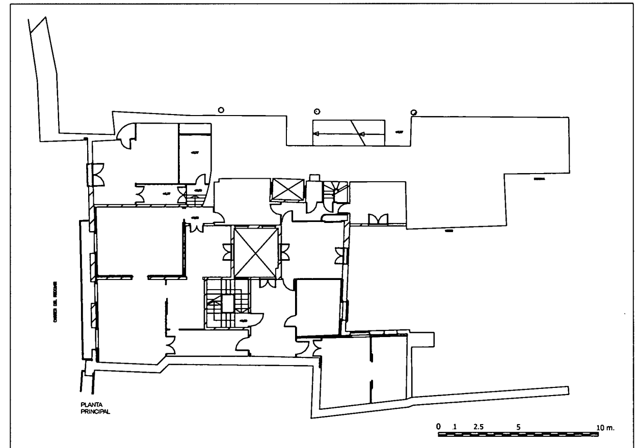
Nivell de planta principal
