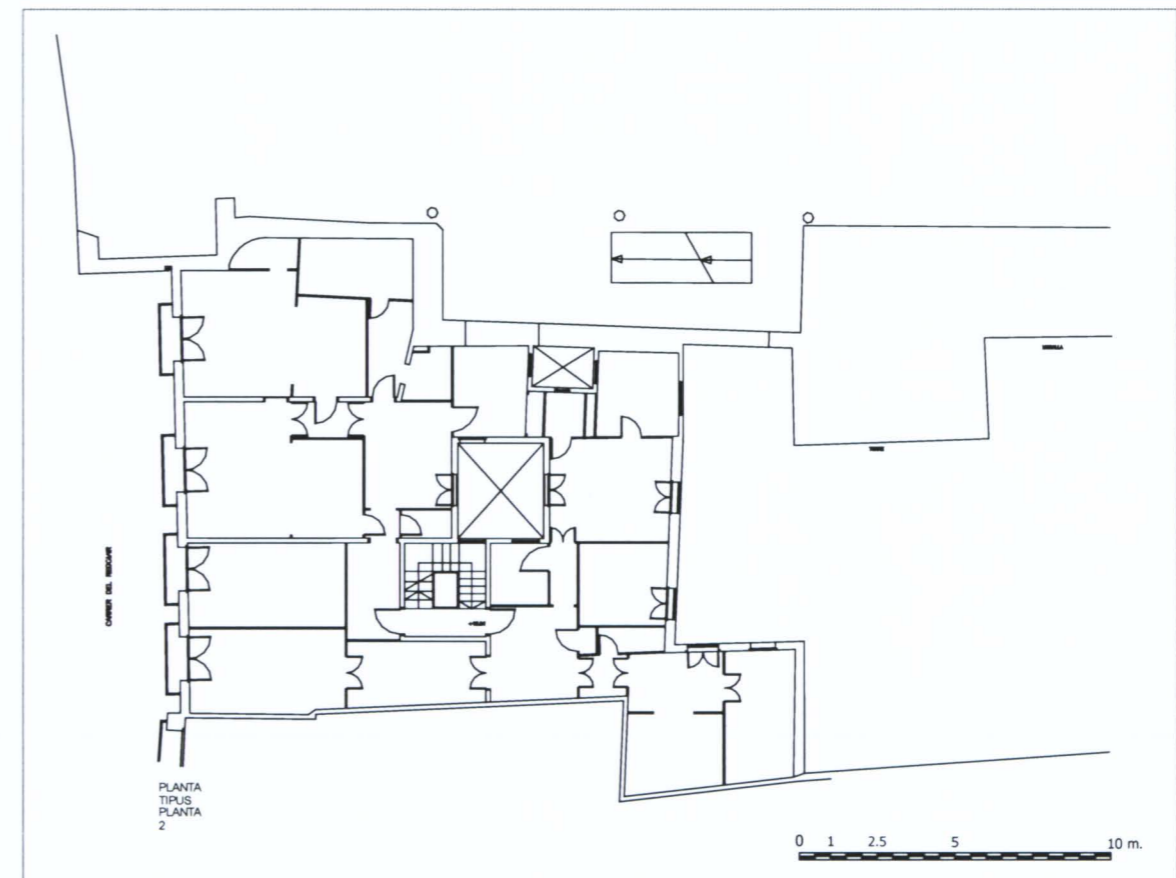
Planta del segon pis de la finca
