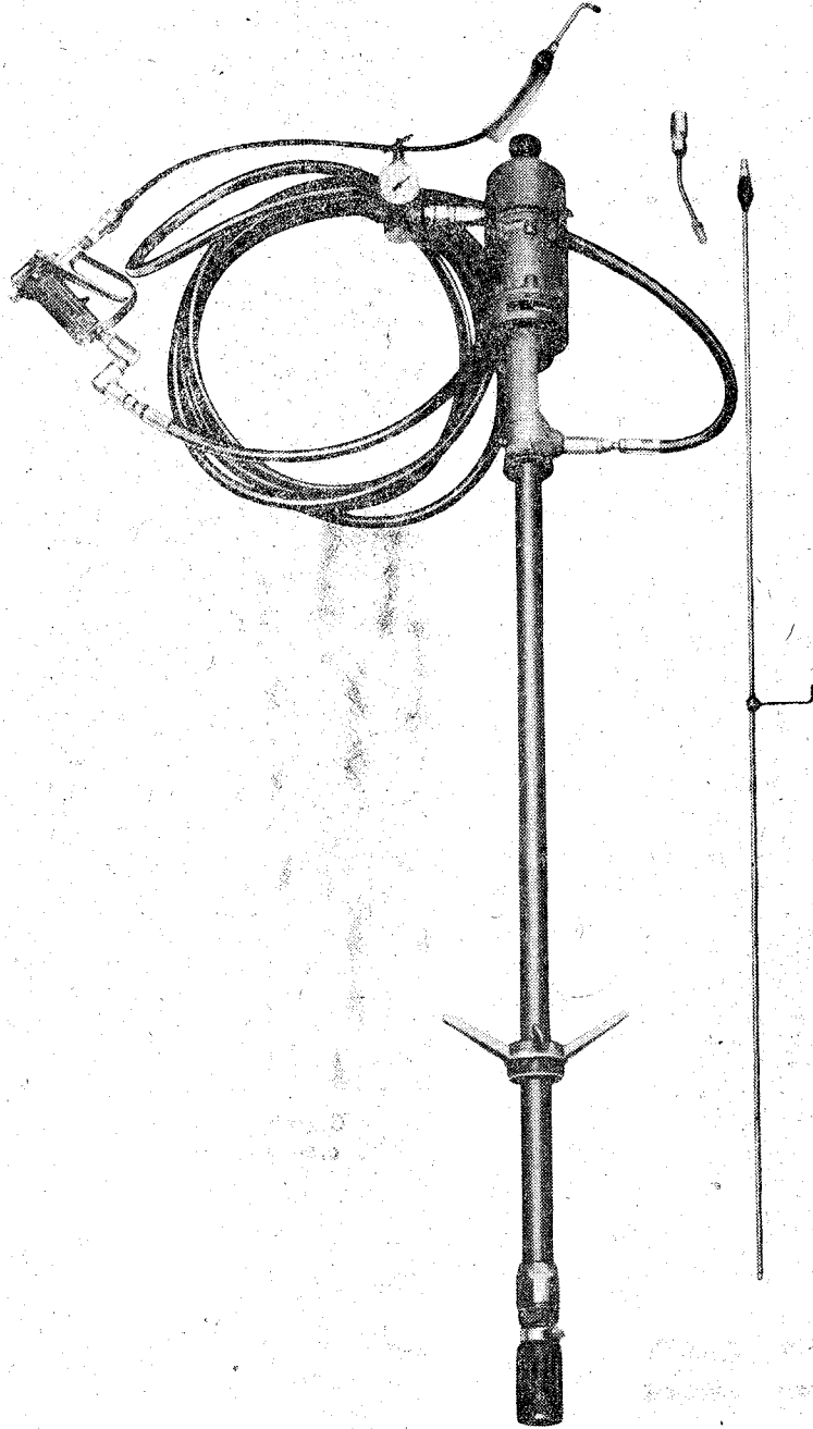
Equipo de pulverización para el tratamiento anticorrosivo Dinitrol, compuesto por bomba de alta presión (Carlese), pistola, boquillas de pulverización y varilla larga.
