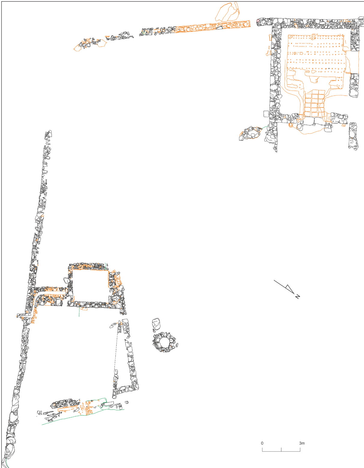
Figura 4. Ca l'Arnau - Can Mateu. Planta del sector del centre productor d'àmfores, 1997-2014
