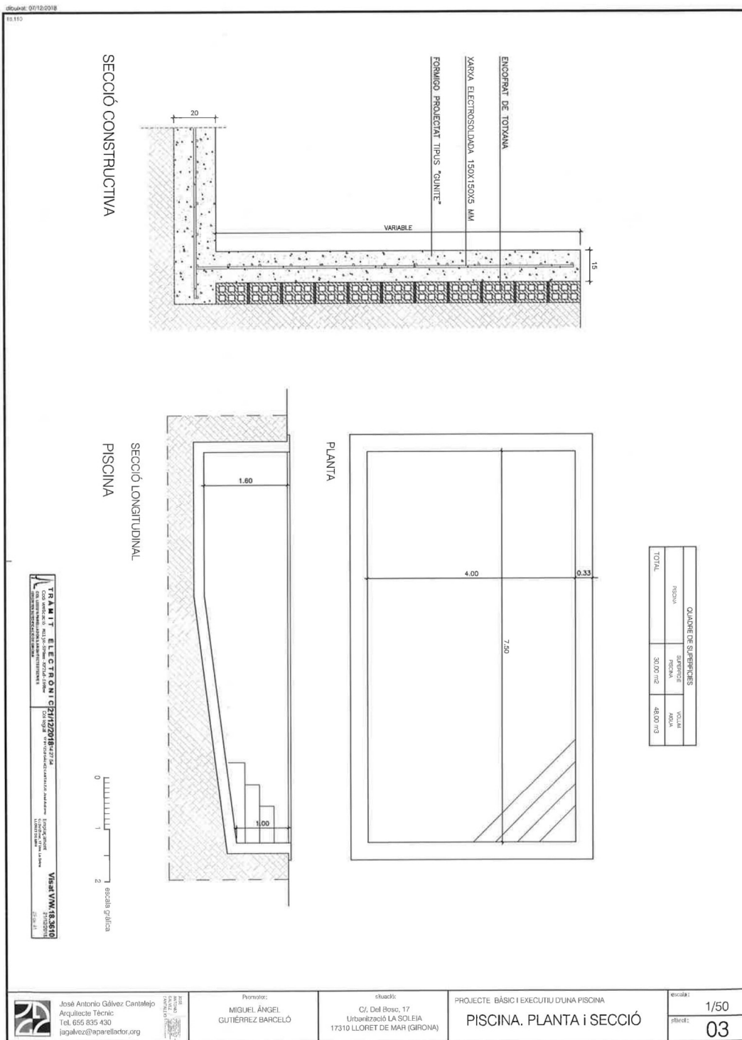
PLÀNOL 5 → Planta i secció de la piscina a construir al carrer del Bosc, 17 Urb. La Soleia (Lloret de Mar), segons el projecte 14 .
