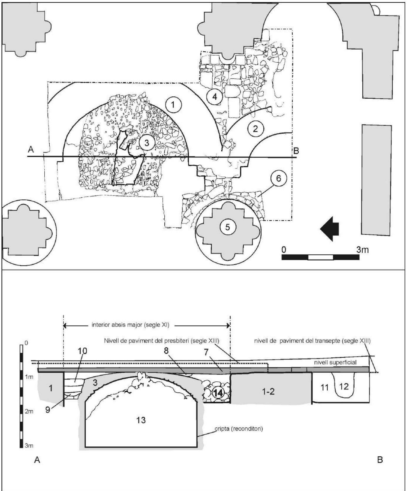
Planta i secciò de la cala núm. 4.
