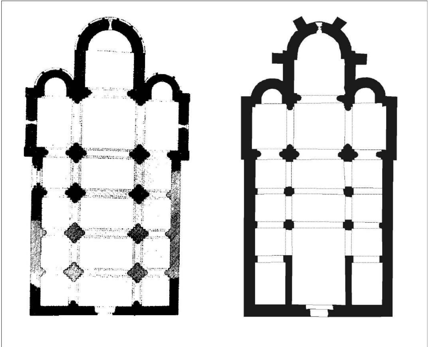
Planta de Santa Maria de Besalú segons Puig i Cadafalch, a l'esquerra, i de Lampérez, a la dreta.
