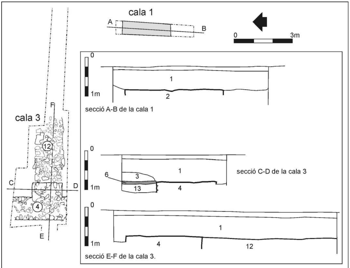
Planta de les cales 1 i 3 i les seccions corresponents.
