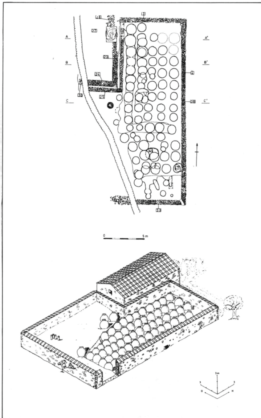
Fig. 1. - Planta de les restes i reconstitució hipotètica del magatzem de l'Olivet d'en Pujol.
