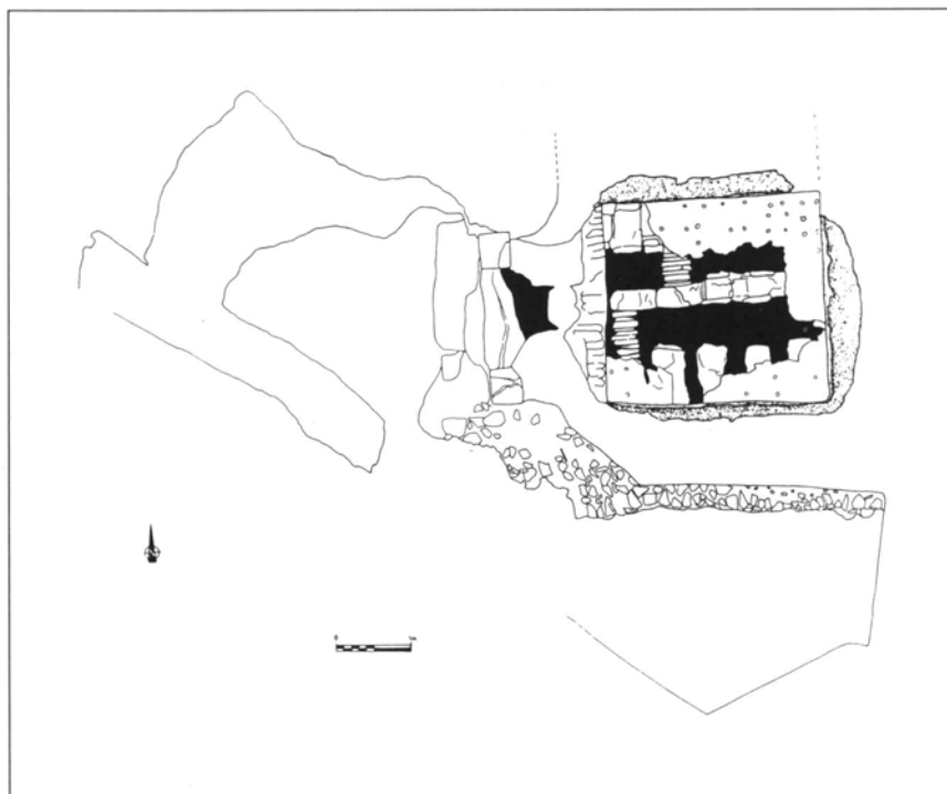
Fig. 1. Planta del forn, amb la cambra anterior i un detall del mur constructiu.
