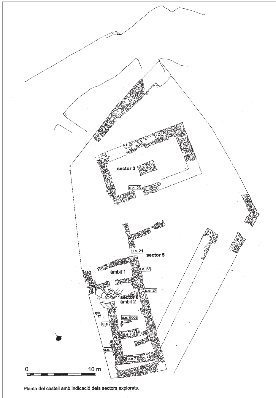
Figura 1. Planta general del castell amb indicació dels sectors excavats.
