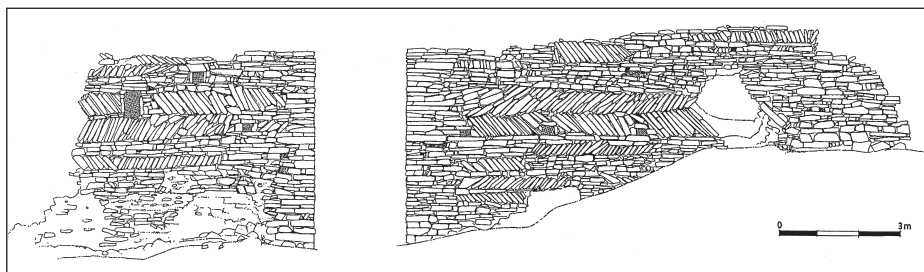
Figura 2. Alçat del parament exterior de les parets nord i est del sector 3 o «torre».
