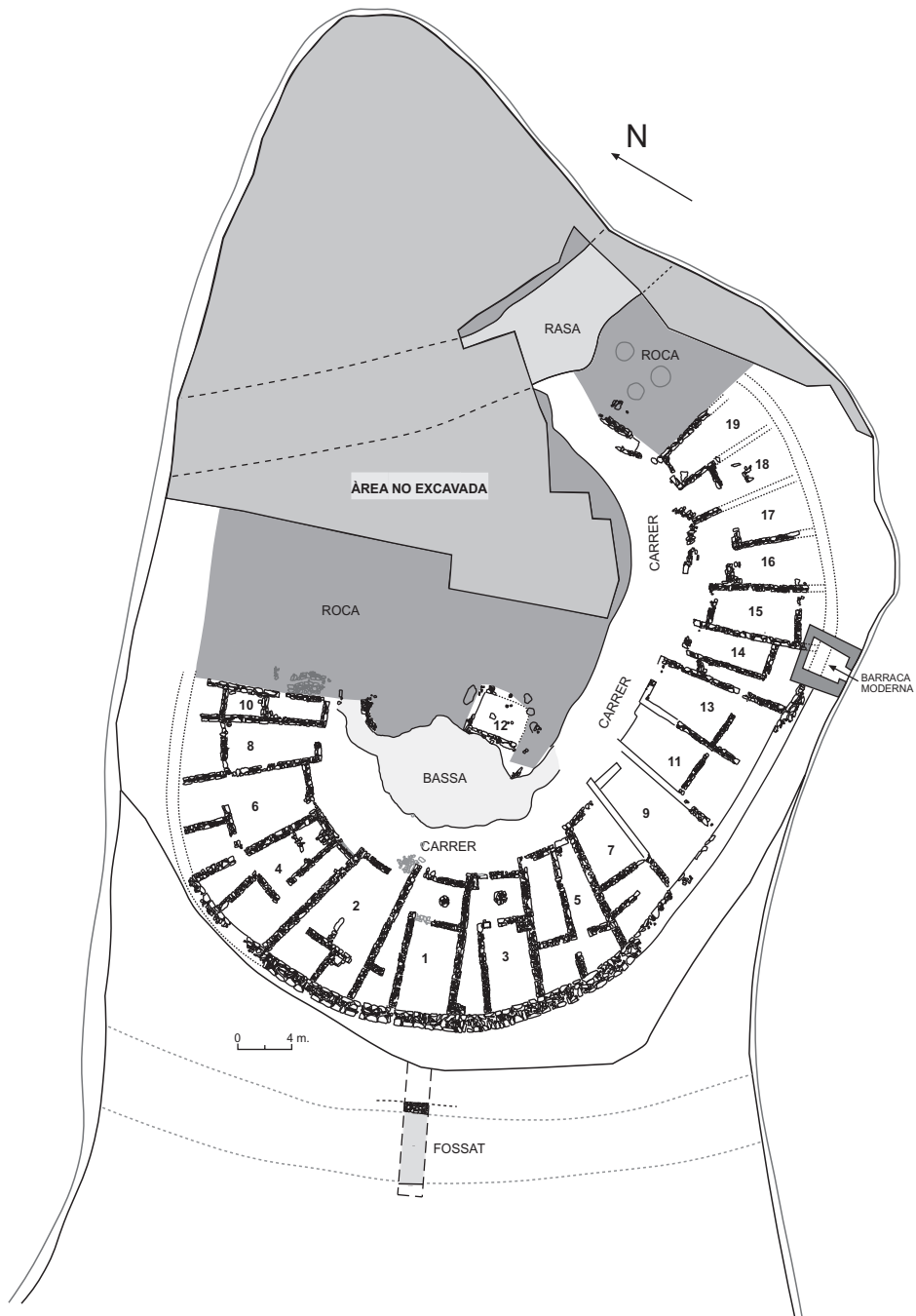
Figura 2. Planta general.
