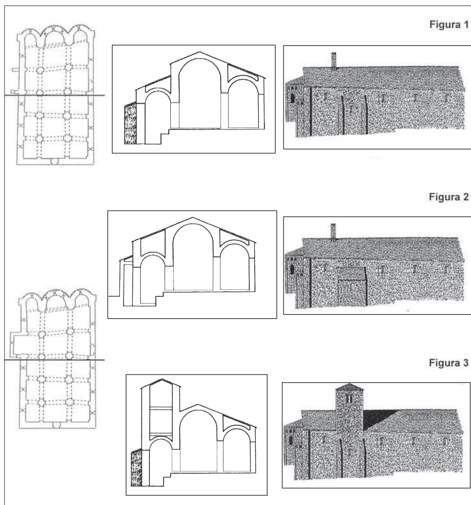
Figura 5. Restitució hipotètica de la planta de l'edifici romànic. Les seccions i els alçats il·lustren diferents propostes d'alçat de la nau lateral nord: amb contraforts (Figura 1) amb capella lateral (Figura 2) i amb campanar (Figura 3).
