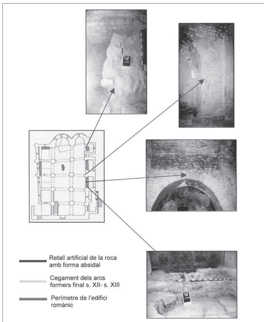
Figura 4. Elements estructurals –identificats mitjançant l'excavació arqueològica i l'estudi de paraments– que permeten restituir el mur de tancament sud de la construcció romànica.
