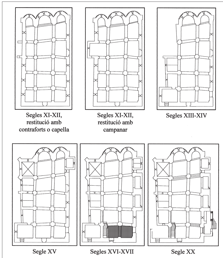
Figura 7. Hipòtesi de l'evolució de la planta de l'edifici.
