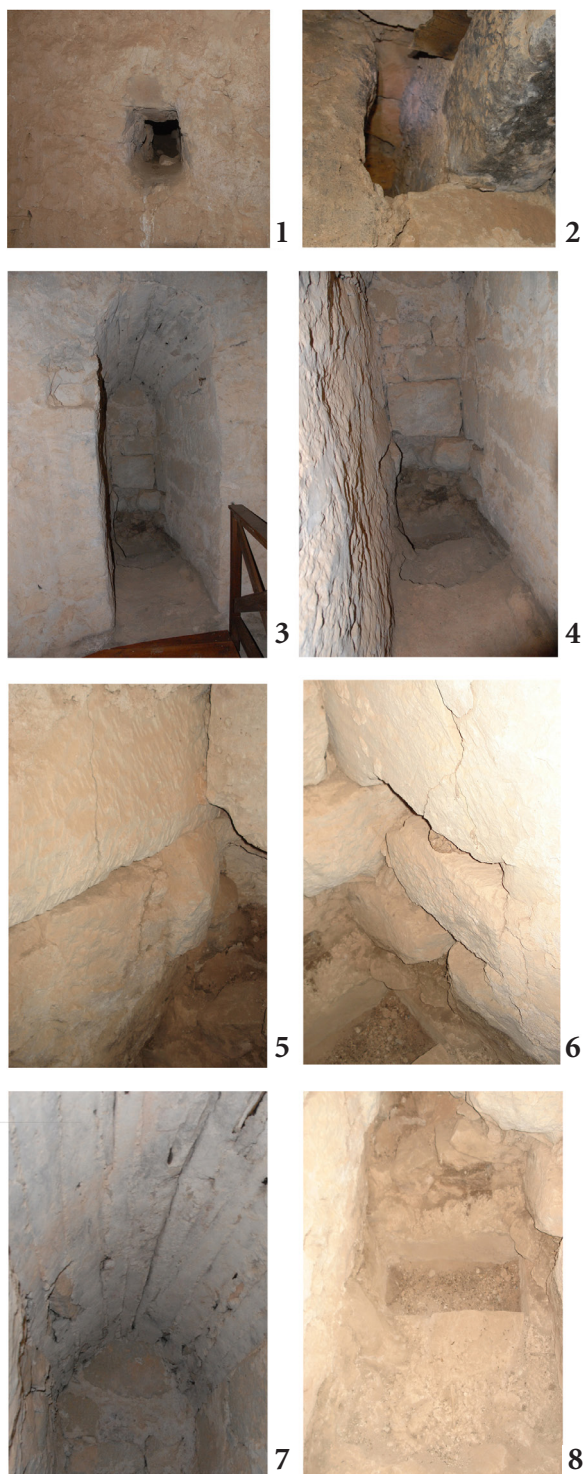
Fig. 7. Llucana de l'anella interior i latrina: 1. llucana des de l'interior de l'anella; 2. des de la xemeneia intramural, sota la segona represa; 3. vista general de la latrina; 4. interior; 5 i 6. encaixos de la taula del seient; 7. volta; 8. albelló
