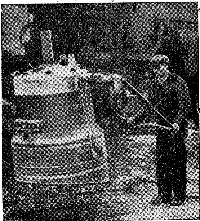
Apisonadora muy empleada en las líneas ferroviarias para la consolidación de las vías. Se le llama «Rena» por los saltos que da al trabajar.—(Calpe)
