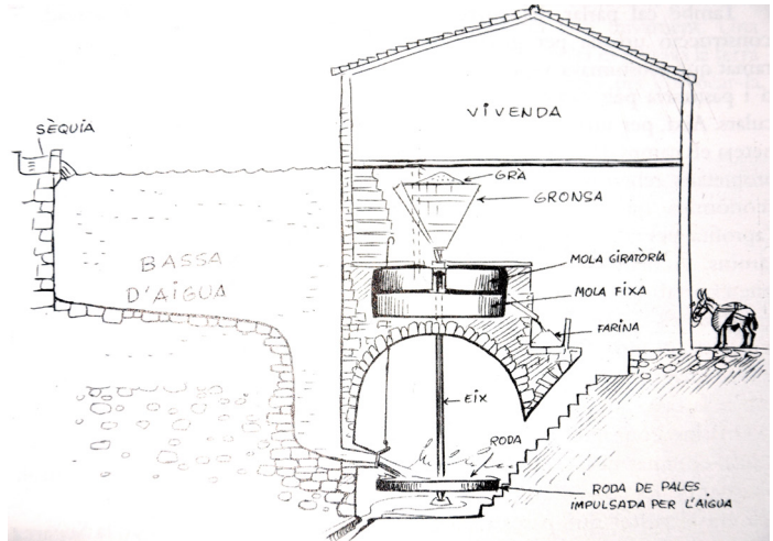
Esquema del molí del Moliner (Carbassers). Dibuix: Francesc Masip.
