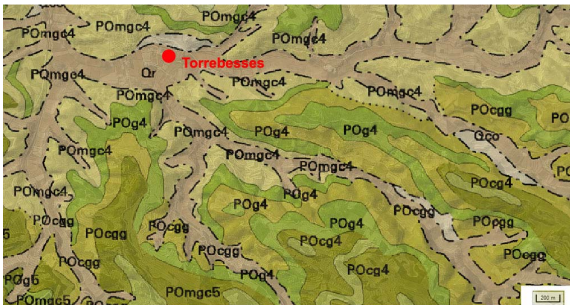
Fig. 1: Mapa geològic 1:50.000 (BG50Mv01r01) de la zona d'estudi superposat a l'ortofotomapa 1:5.000 (OF-5M v6.0).
