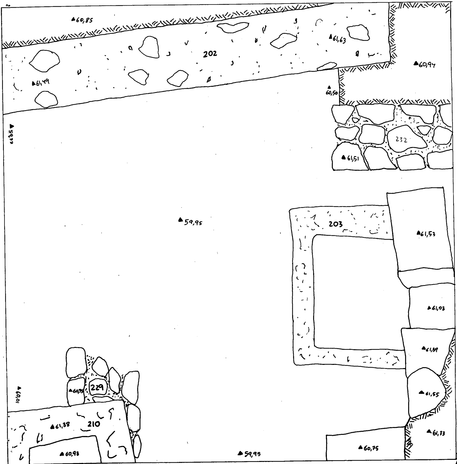
PLAÇA DELS ANGELS PLANTA SONDEIG 200 ESCALA 1/20 COTES ESTRUCTURES I ROCA
