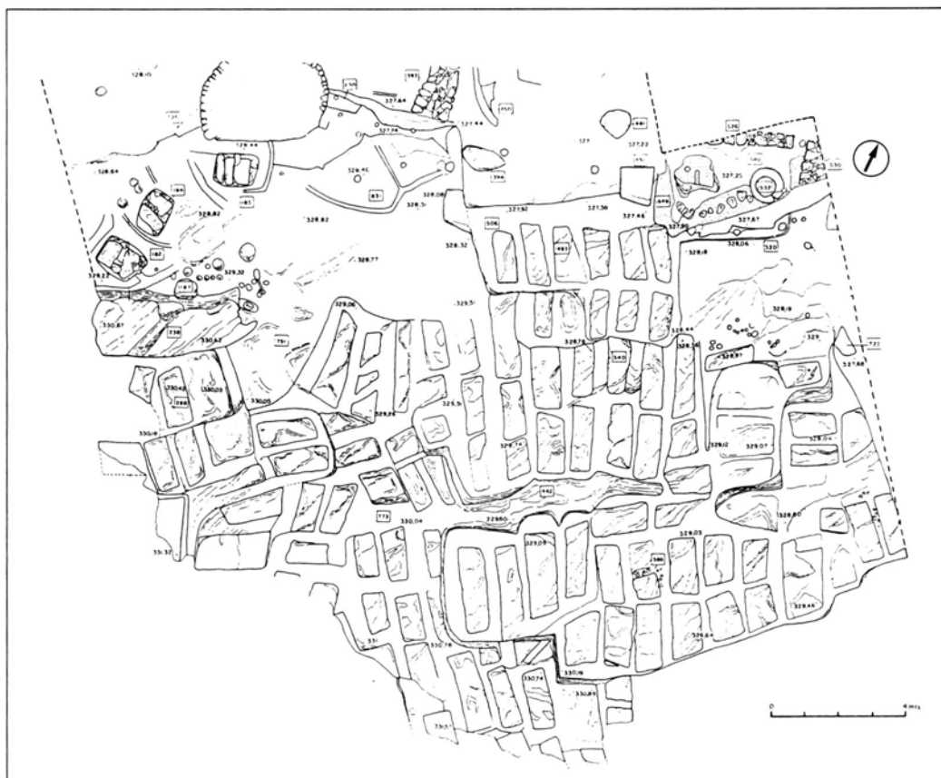
Fig. 4. Planta de la pedrera interior (campanya de 1989).
